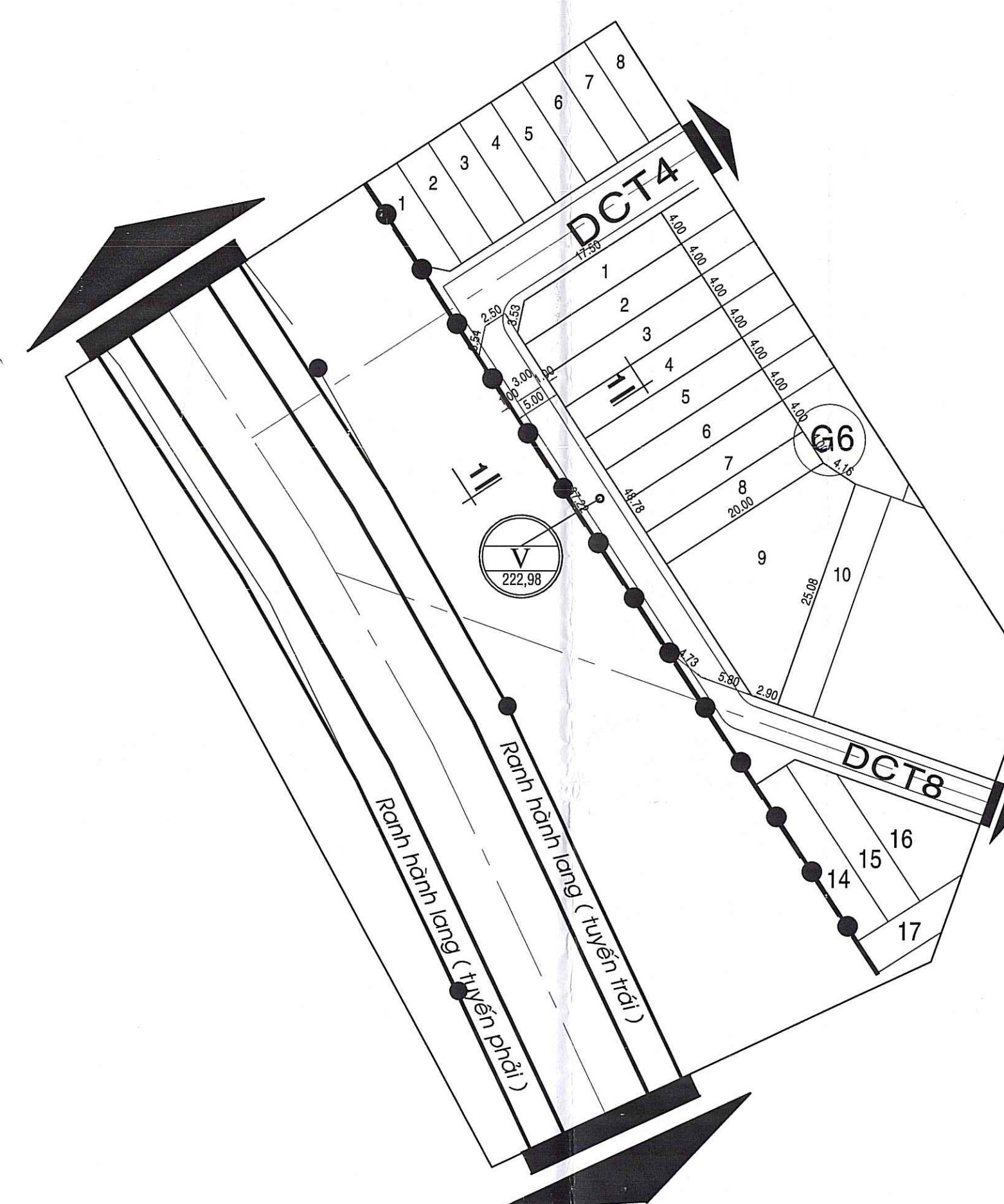
BẢN ĐỒ QUY HOẠCH GIAO THÔNG ĐÔ THỊ & CHỈ GIỚI ĐƯỜNG ĐỎ, CHỈ GIỚI XÂY DỰNG
