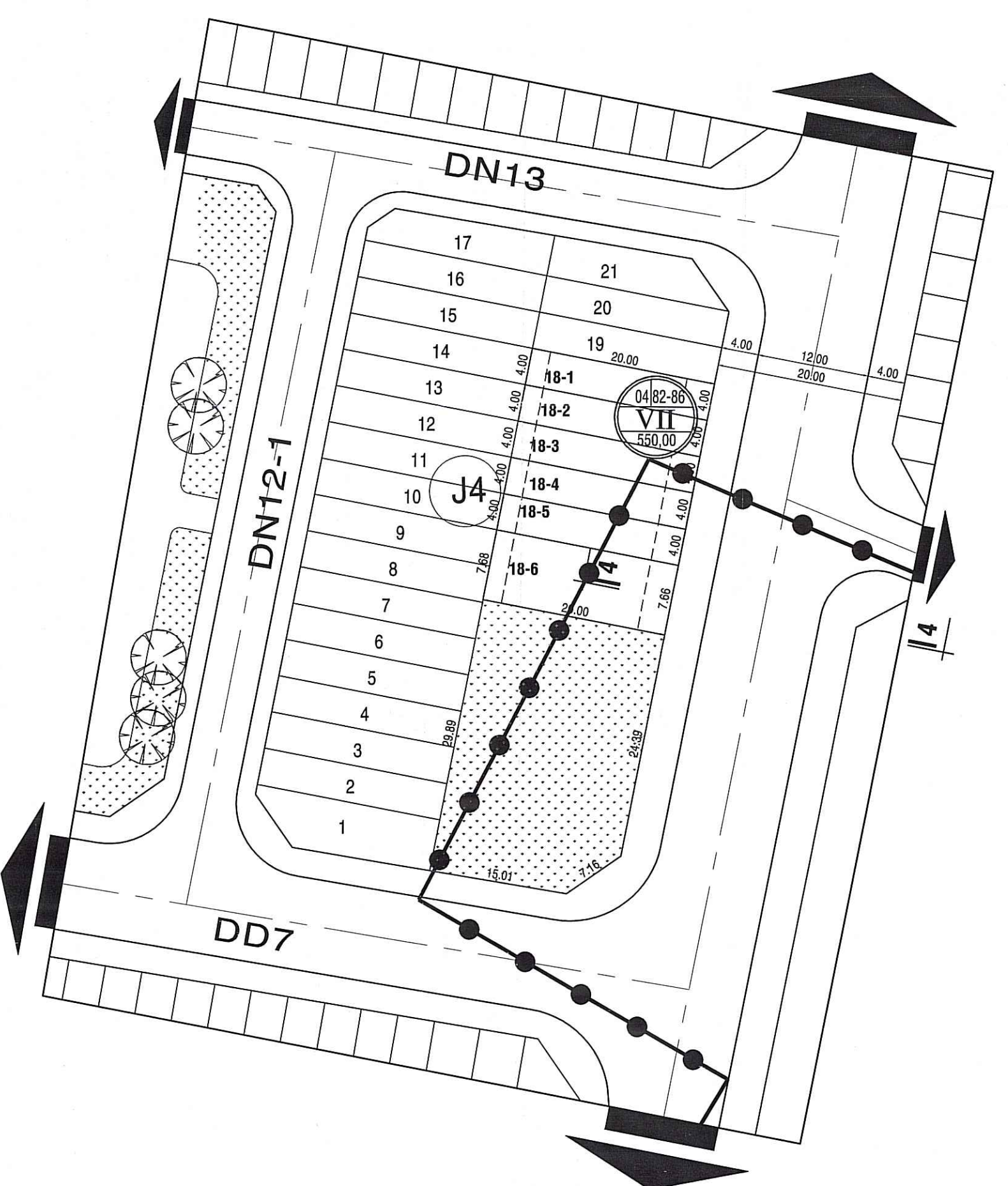
BẢN ĐỒ QUY HOẠCH GIAO THÔNG ĐÔ THỊ & CHỈ GIỚI ĐƯỜNG ĐỎ, CHỈ GIỚI XÂY DỰNG
