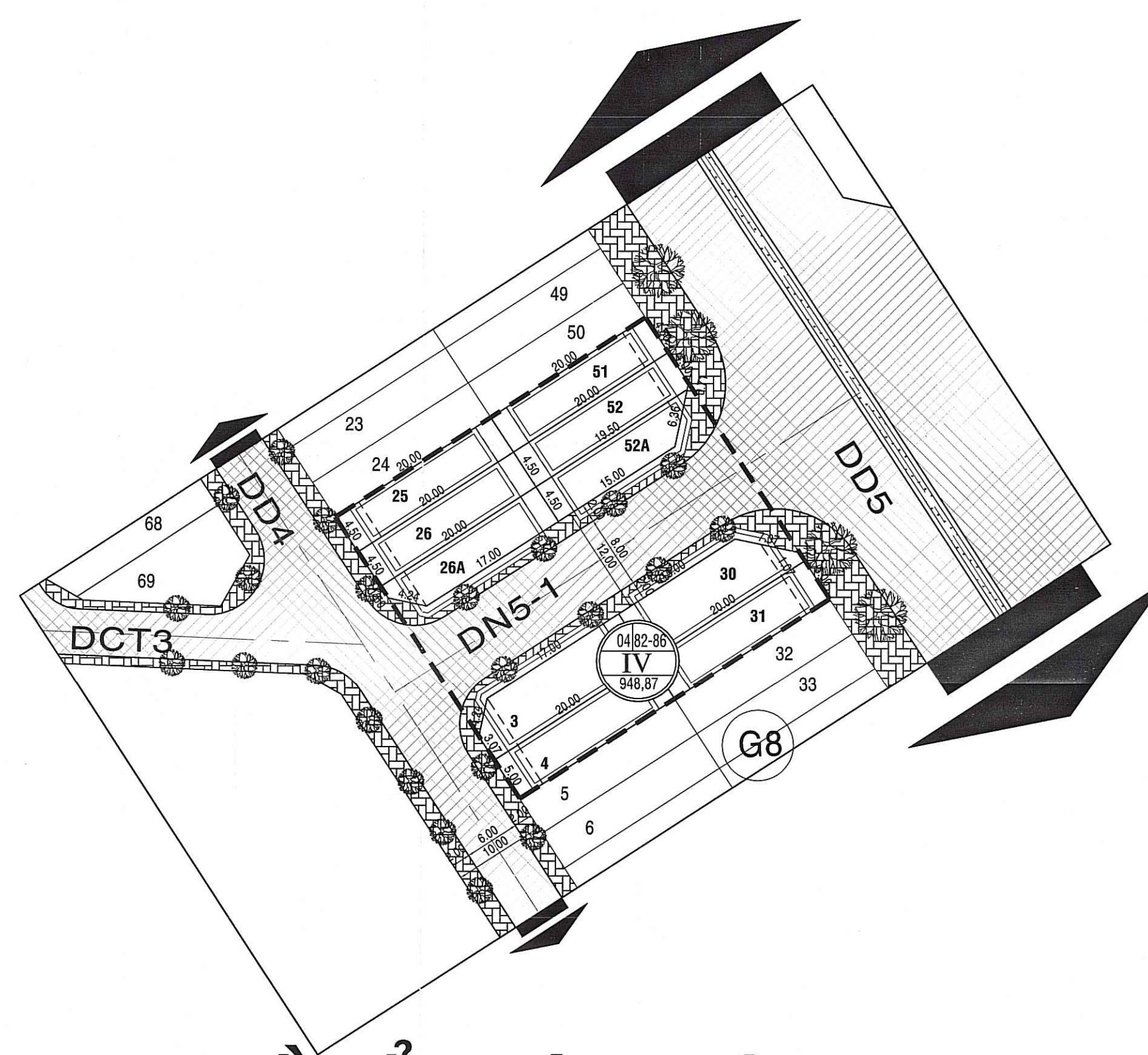
SƠ ĐỒ TỔ CHỨC KHÔNG GIAN KIẾN TRÚC, CẢNH QUAN ĐIỀU CHỈNH
